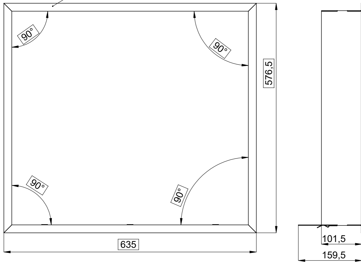
POHLEDOVÁ STRANA
