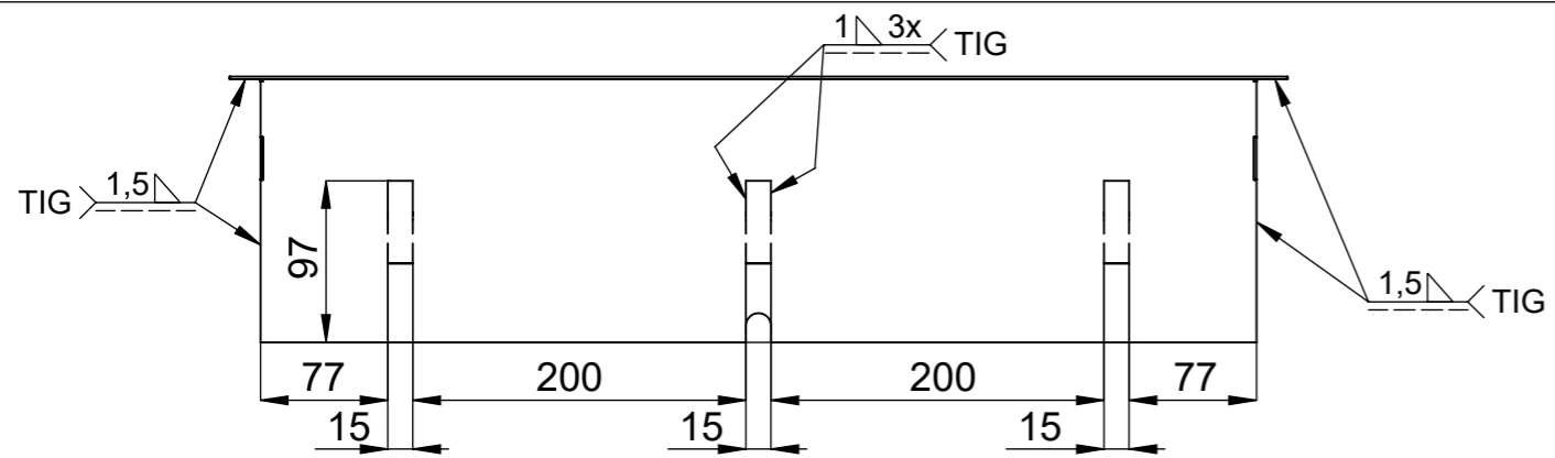
POHLEDOVÁ STRANA
